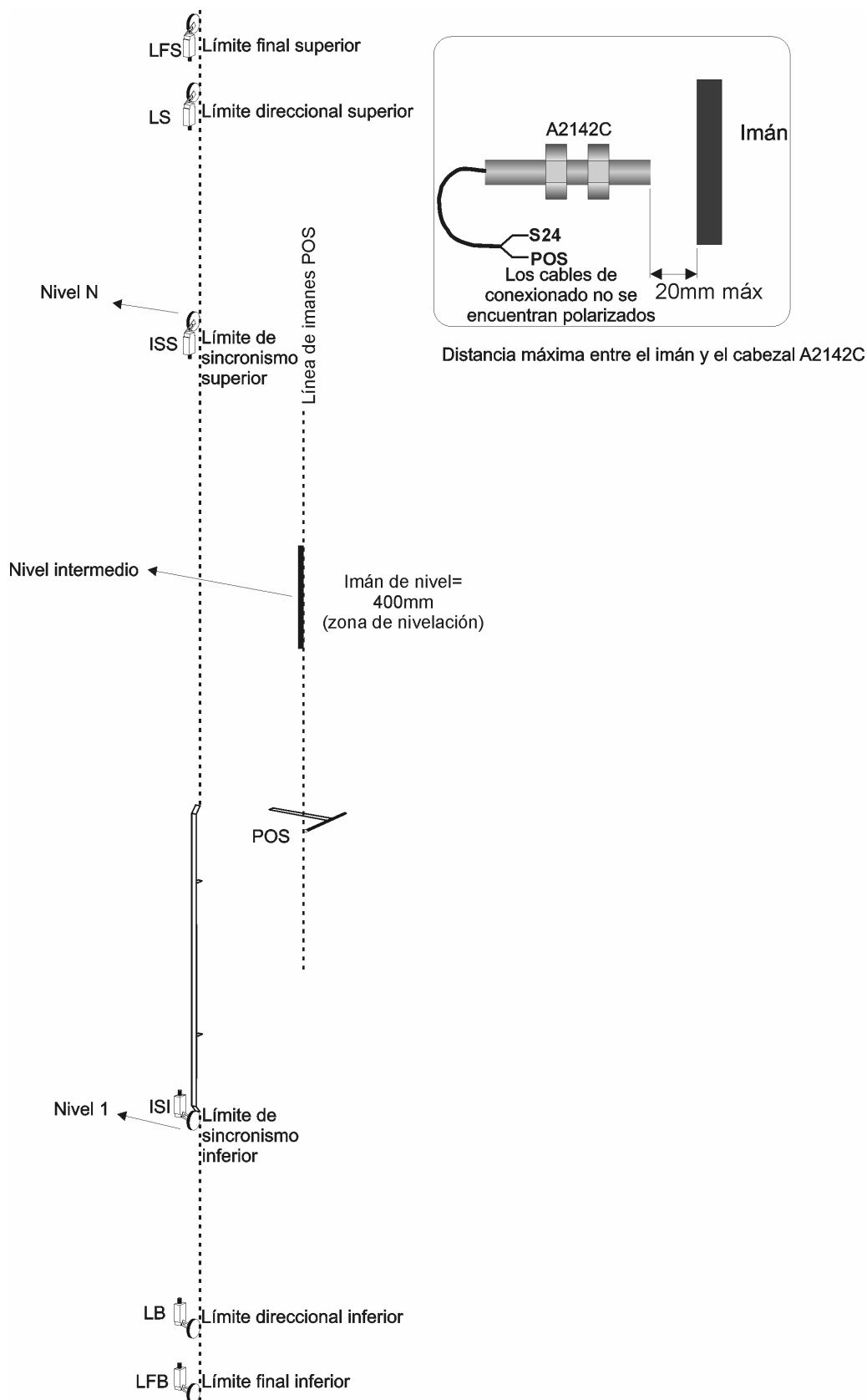
Ilustración 5: Distribución de imanes y límites en el hueco con cabezal magnético tipo lápiz A2142C
