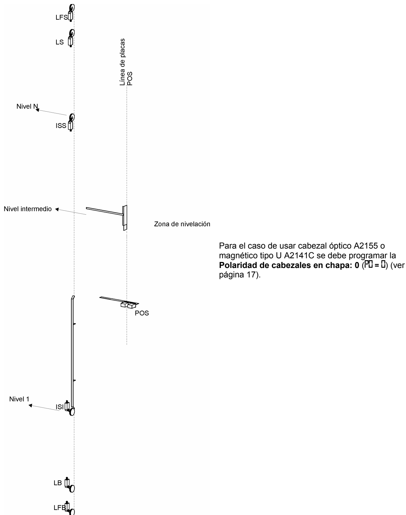
Ilustración 4: Distribución de placas y límites en el hueco con cabezal óptico A2155 o magnético tipo U A2141C
